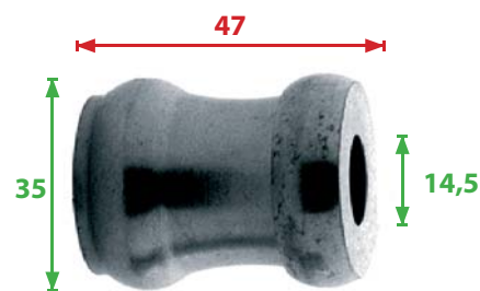
OPEN SPACING SPOOL ENTRETOISE OUVERTE ABSTANDSHALTER OFFEN
