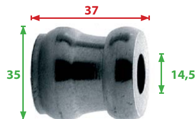
CLOSED SPACING SPOOL ENTRETOISE FERMEE ABSTANDSHALTER GESCHLOSSEN
